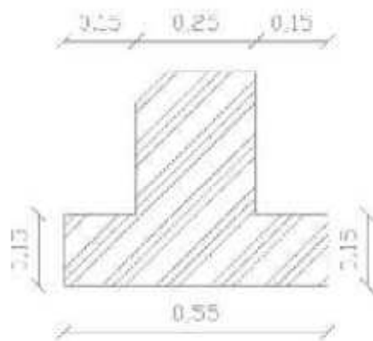
Εικόνα: Διατομή κρασπέδου που τοποθετείται στην περίμετρο της στρώσης διαβαθμισμένων βότσαλων
