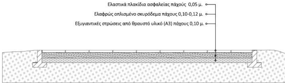
Εικόνα: Διατομή ενδεικτικής εφαρμογής δαπέδου ασφαλείας
