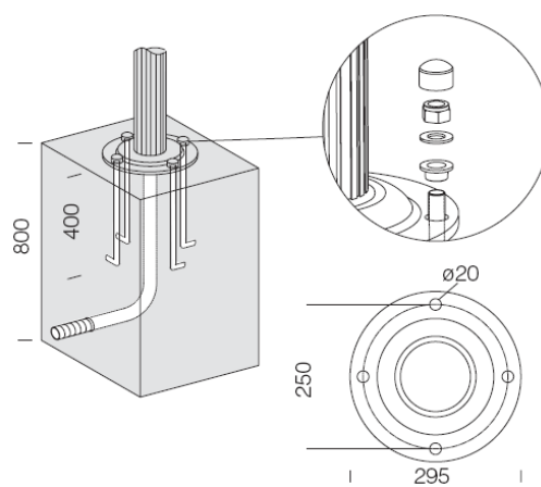
Ενδεικτικό Σκαρίφημα βάσης σύνδεσης
