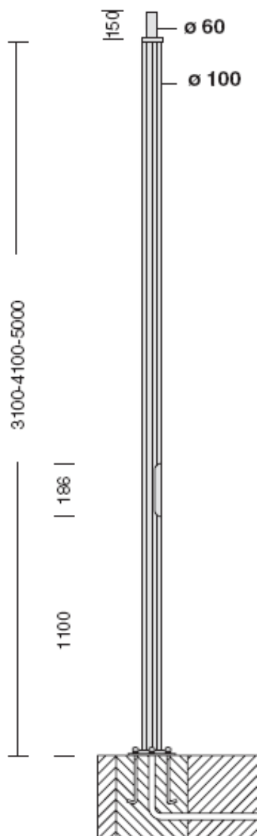
Ενδεικτικό Σκαρίφημα στύλου
