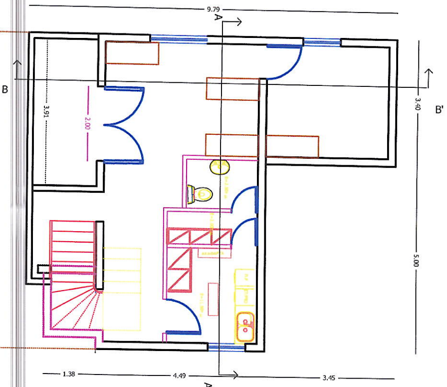
Προτεινόμενη κάτοψη 1ου ορόφου
