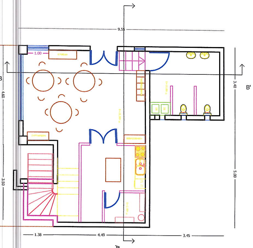
Προτεινόμενη κάτοψη 1ού ορόφου
